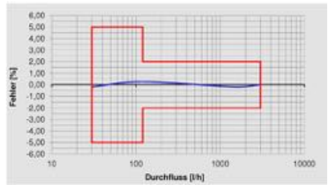
Tipik hata Eğrisi Qn 1,5 sınıf B
